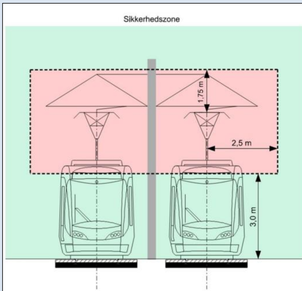
Figur 1 – Den røde felt illustrerer Letbanens sikkerhedszone, hvor høje genstande i form af stiger, lifte, stilladser mm ikke er tilladt.
