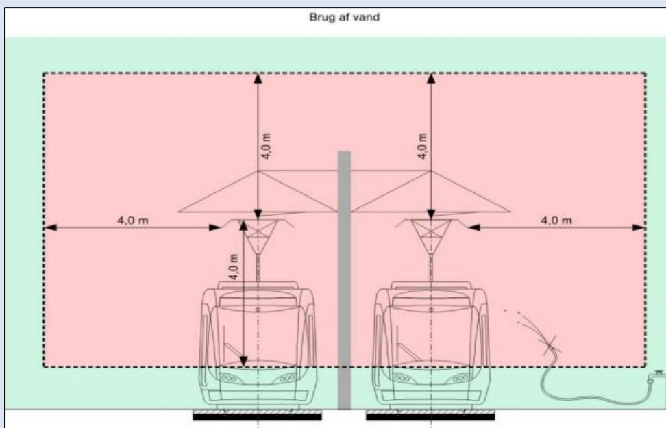
Figur 2 - Brug af vand i nærheden af letbanen er ikke tilladt, hvis vandstrålen peger ind mod letbanen og de strømførende dele.
