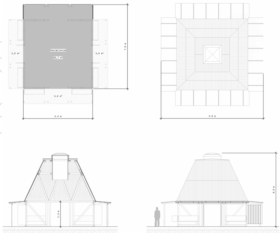
Figur 3. Plan, facader og snit af informationspavillon.
