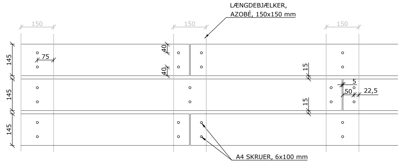
DETALJE, PRINCIP FOR SAMLINGER VED DÆKPLANKER OG LÆNGDEBJÆLKER TRÆDÆK VED POLOMRÅDE (1:10)
